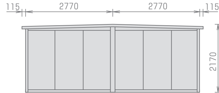
【A立面図】
