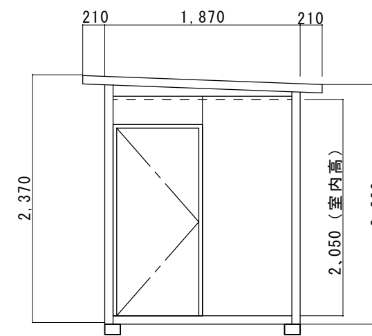
【D立面図】
