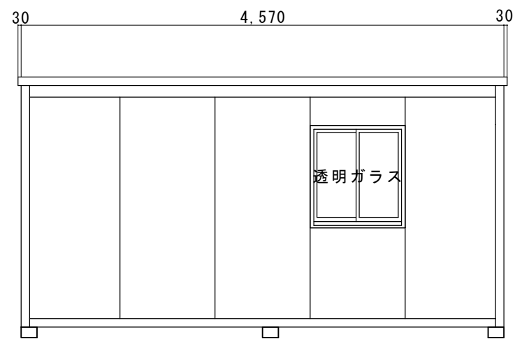
【A平面図】
